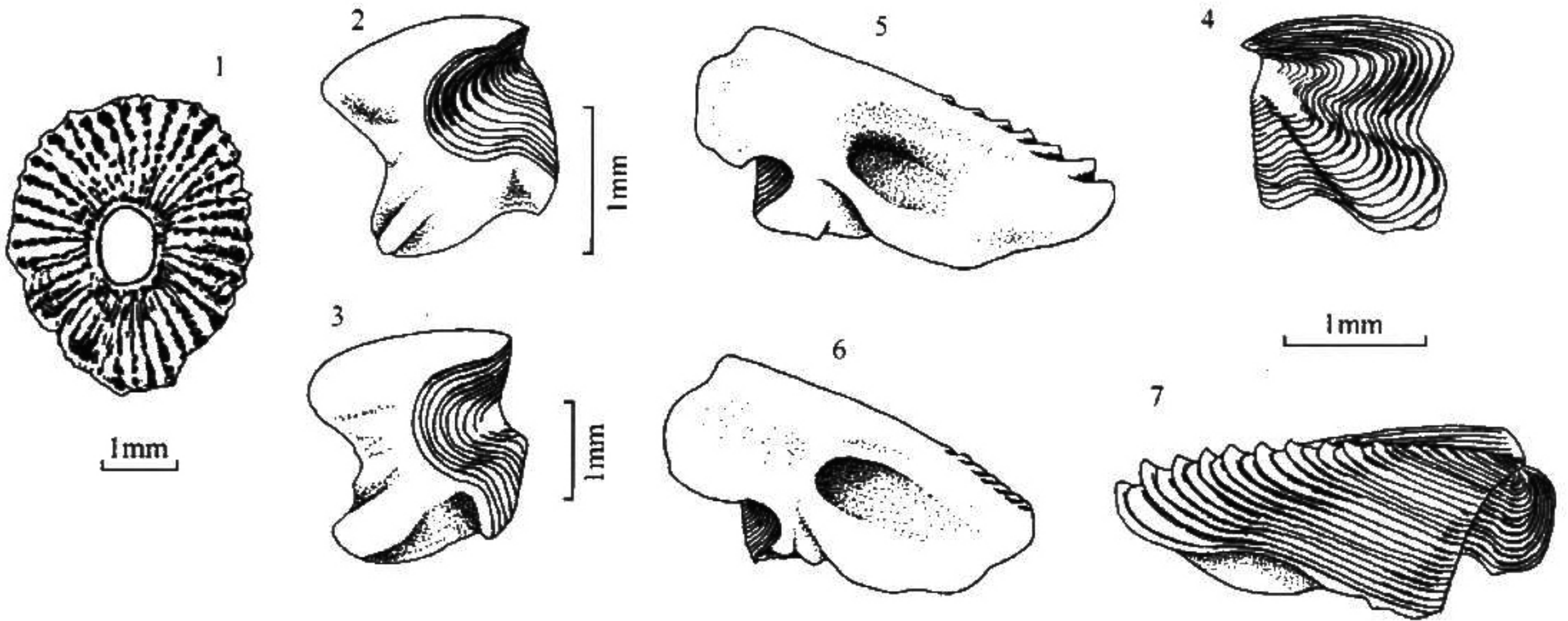
图 209 东方宽楯藤壶 Savignium orientale Ren 1. 外形; 2~4. 背板; 5~7. 楯板
