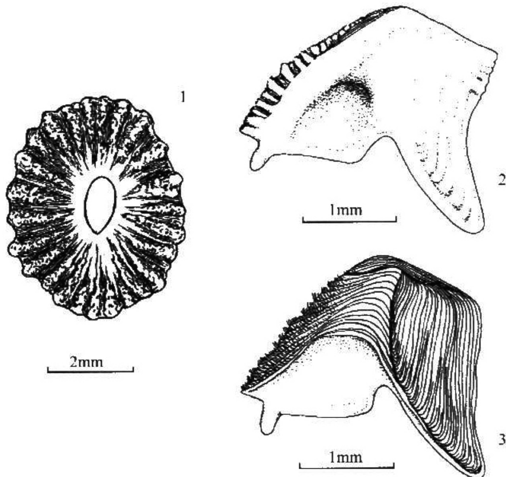
图 210 连贵藤壶 Nobia conjugatum (Darwin)
